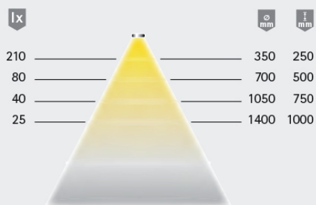
Diagrama de distribución luminosa / 70° (longitud 600 mm)
